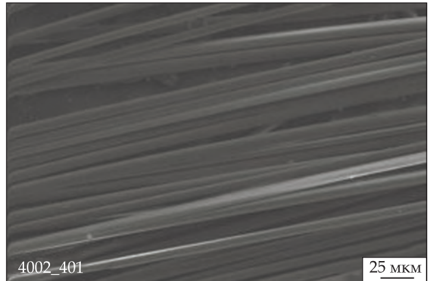
Структура базальтової комплексної нитки — ровінгу
