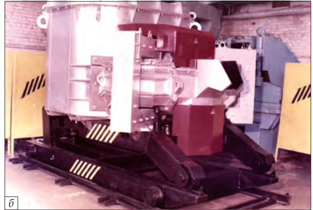
Магнітодинамічні міксери-дозатори для алюмінієвих сплавів (а), для чавуну і сталі (б)
