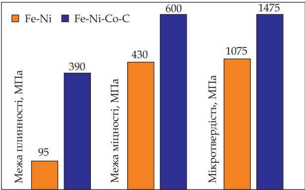
Залежність межі плинності, межі міцності та мікротвердості інварних сплавів на основі Fe-Ni: помаранчеві колонки — стандартний сплав; фіолетові колонки — пропонується інварний сплав
