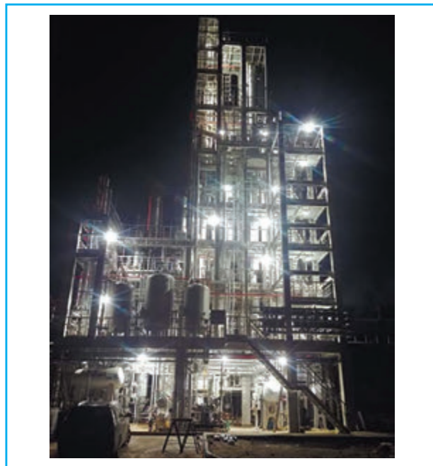
НРРОа установка з виробництва пропіленоксиду на ТОВ «Карпатнафтохім»
