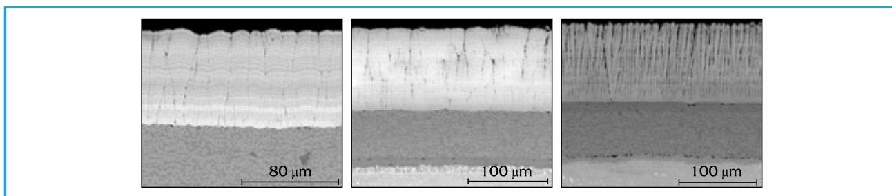
Мікроструктури покриттів з верхнім керамічним шаром: а – ZrO_2 – ЛК; б – ZrO_2 – ВК; в – ZrO_2 – Y_2O_3
