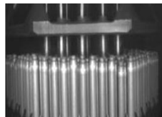
Візуальний контроль ТВЗ-WR після кожного року експлуатації
