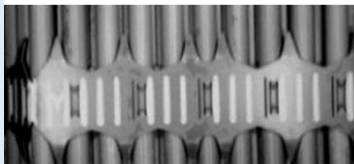
Візуальний контроль ТВЗ-WR після кожного року експлуатації
